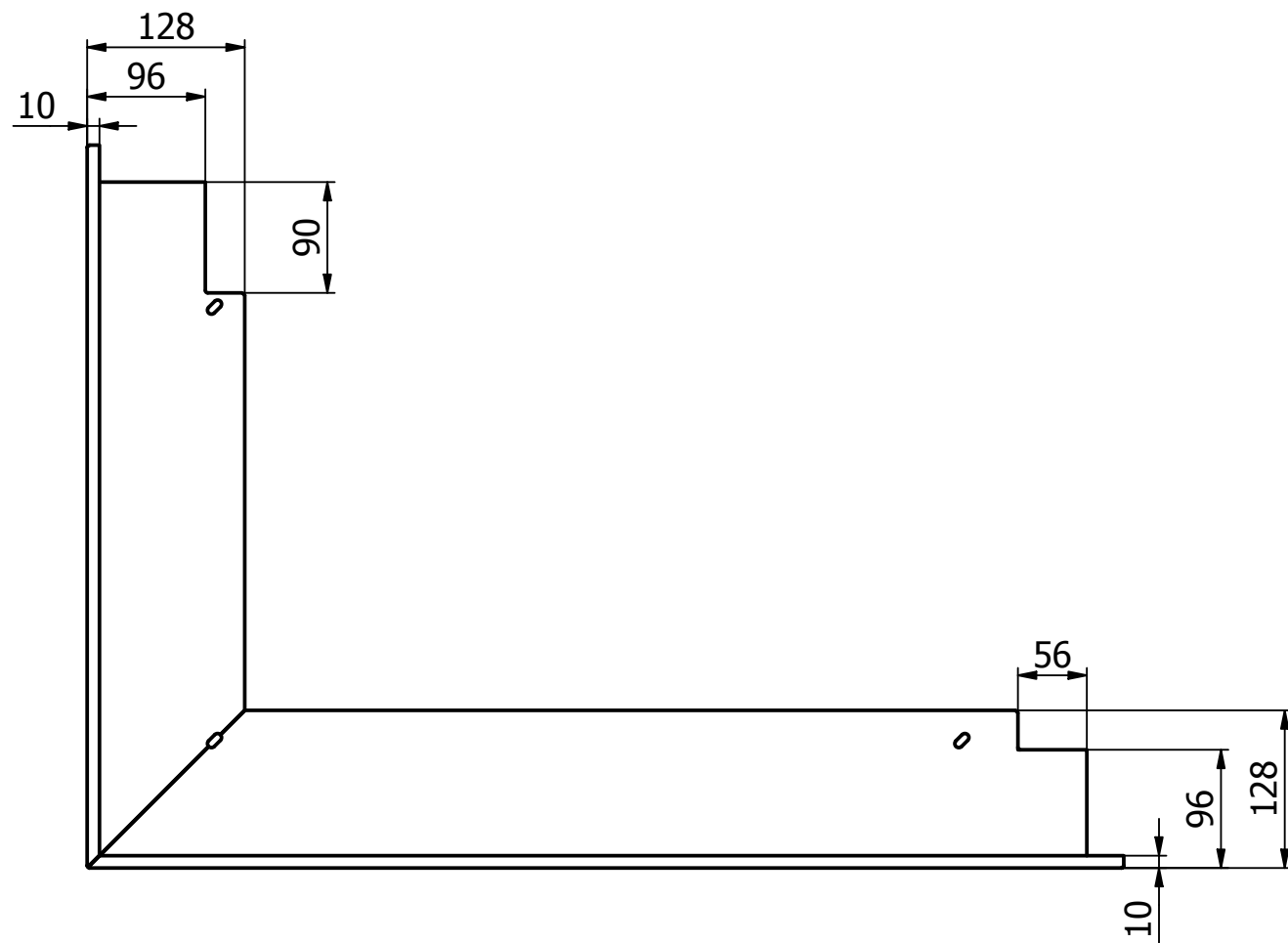
Maskownica 30 głęboka
